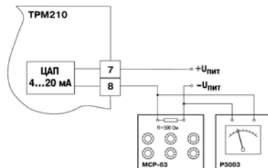
Рисунок Ж.5 – Подключение ВУ2 типа И
