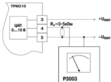
Рисунок Ж.6 – Подключение ВУ1 типа У
