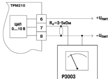
Рисунок Ж.7 – Подключение ВУ2 типа У
