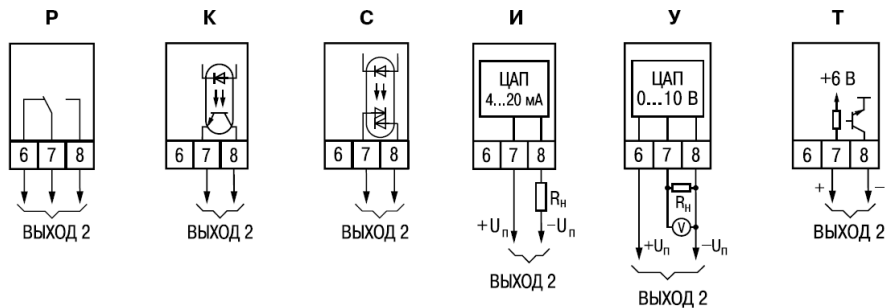
Рисунок Б.4 – Схемы подключения к различным модификациям ВУ2
