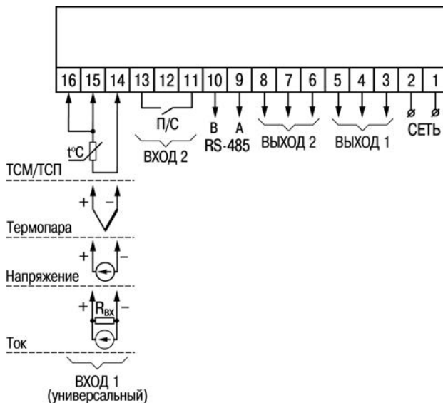
Рисунок Б.2 – Общая схема подключения TRM210-H2
