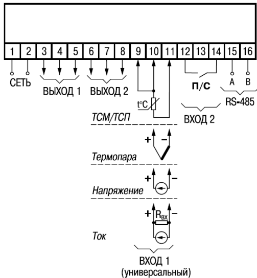
Рисунок Б.1 – Общая схема подключений TRM210-Н, Щ1 и Щ2
