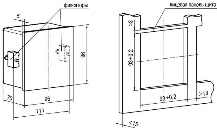
Рисунок А.3 – Прибор щитового крепления Щ1
