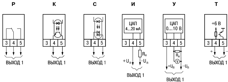
Рисунок Б.3 – Схемы подключения к различным модификациям ВУ1
