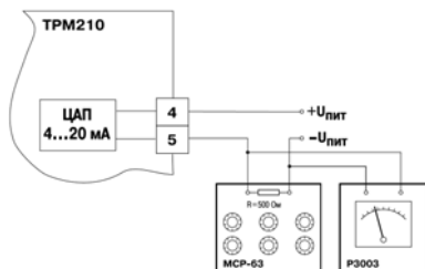
Рисунок Ж.4 – Подключение ВУ1 типа И
