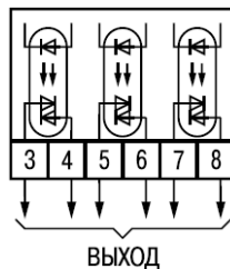
Рисунок Б.5 – Схема подключения ОВЕН ТРМ210-Х.С3
